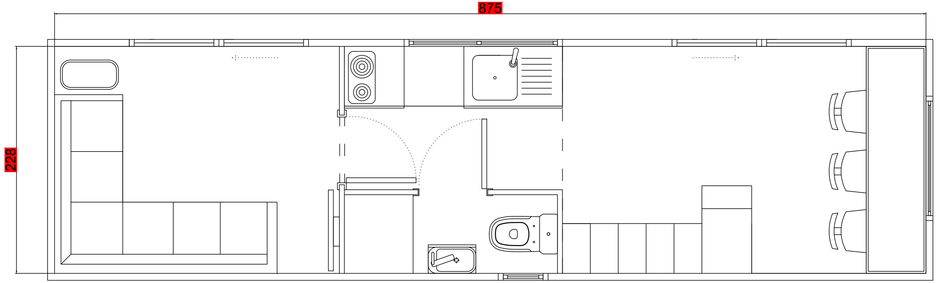
ZEMİN KAT YERLEŞİM PLANI
